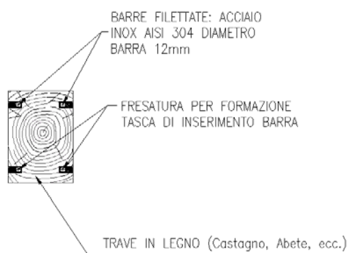
Figura 99. Ricostruzione dell'estremità di trave in legno appoggiata alla parete muraria mediante protesi di testata: a) sezione longitudinale; b) sezione trasversale
