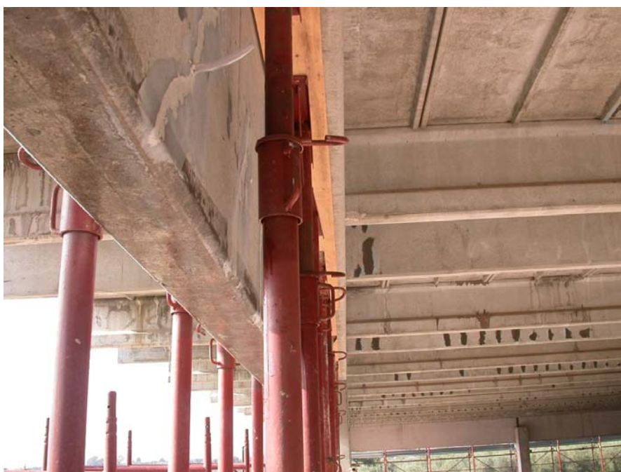
Figura 80. Rinforzo a flessione con compositi di una trave in c.a.
