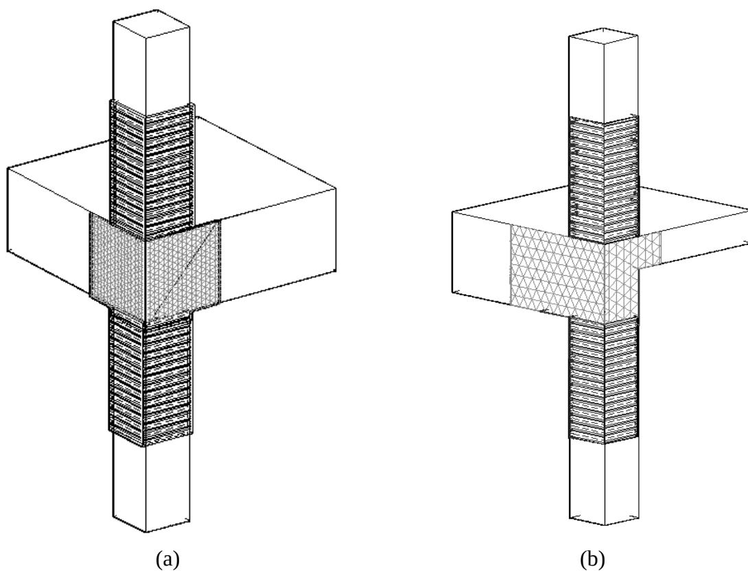
Figura 36. Confinamento di pilastri di un nodo d'angolo: (a) nodo con due travi emergenti; (b) nodo con una trave emergente ed una a spessore
