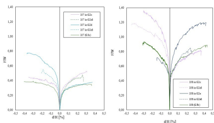
Curve forza – spostamento normalizzate sul peso dell'edificio (US)
