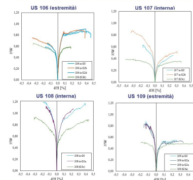
Curve forza – spostamento normalizzate sul peso dell'edificio (US)
