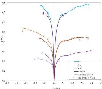
Curve forza – spostamento normalizzate sul peso dell'aggregato (G0)
